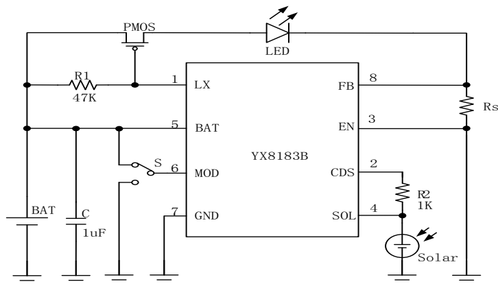
图 4 方案二：PMOS 扩流方案
