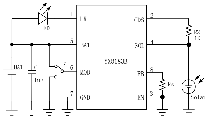
图 3 方案一：直驱方案
