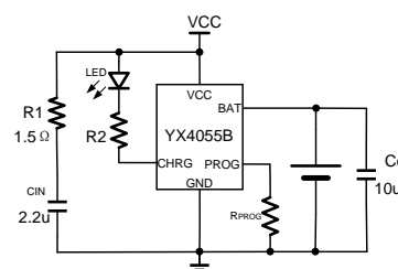
图 1. 典型应用电路
