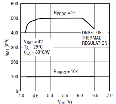
充电电流 vs 电源电压
