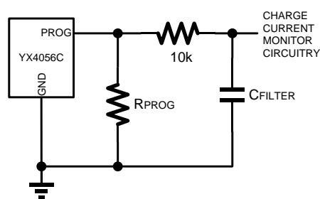
图3 隔离PROG引脚上的容性负载和滤波器
