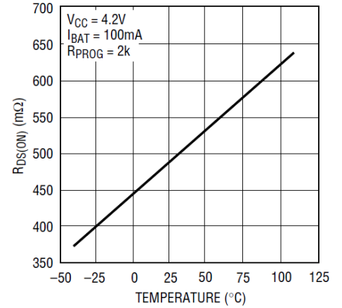
功率 MOS 开态电阻 vs 温度
